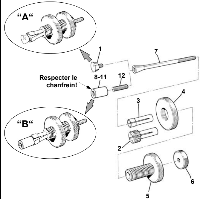
Fig. 2: Assembler l'outil de centrage d'embrayage.
