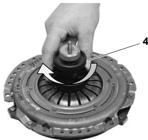
Fig. 5: Monter le disque d'embrayage.
