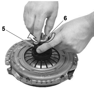
Fig. 3: Placer l'outil de centrage d'embrayage en l'insérant sur les écrous de serrage.
