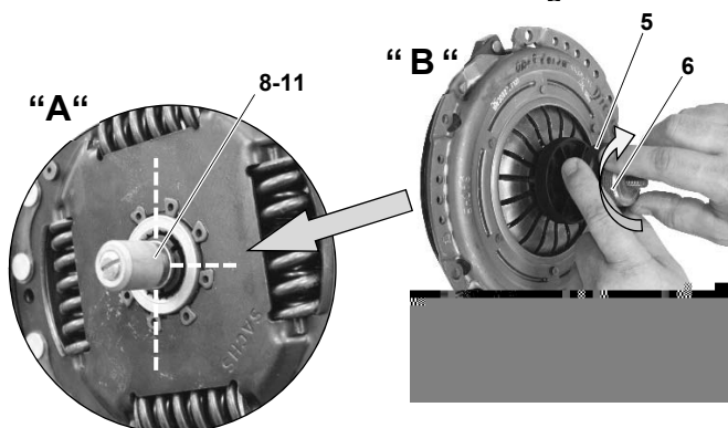
Fig. 8: Serrer légèrement l'écrou de blocage sur la plaque de pression.
