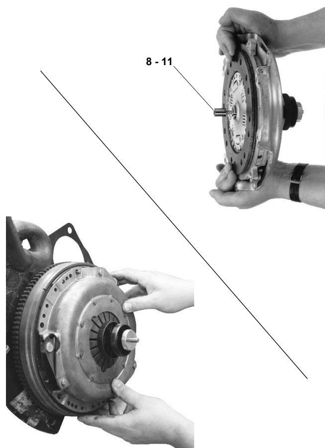
Fig. 9: Monter la plaque de pression avec le disque d'embrayage sur le volant moteur selon les instructions du constructeur.
