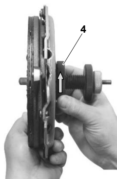
Fig. 9: Monter la plaque de pression avec le disque d'embrayage sur le volant moteur selon les instructions du constructeur.
