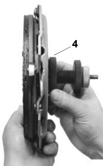
Fig. 6: Serrer l'écrou de blocage.
