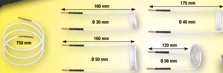
500.8605 Set de pistolets à chaleur par induction
